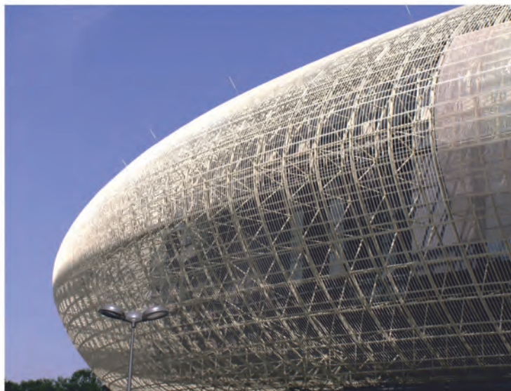
Maszt izolowany mocowany do konstrukcji hali sportowo-widowiskowej w celu ochrony ekranu LED.
